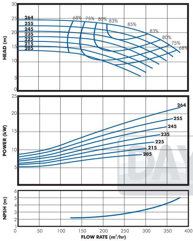
MODEL DE 125/40
