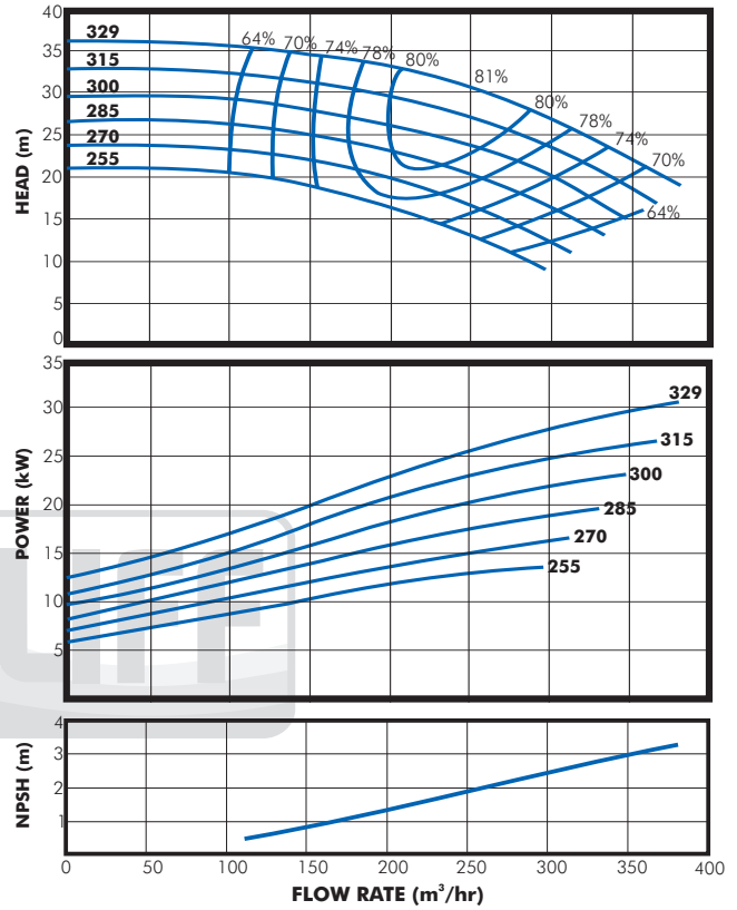
MODEL DE 125/32
