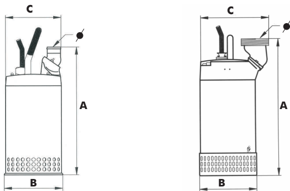
DW50.08.3
