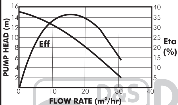
DW.50.08.03
